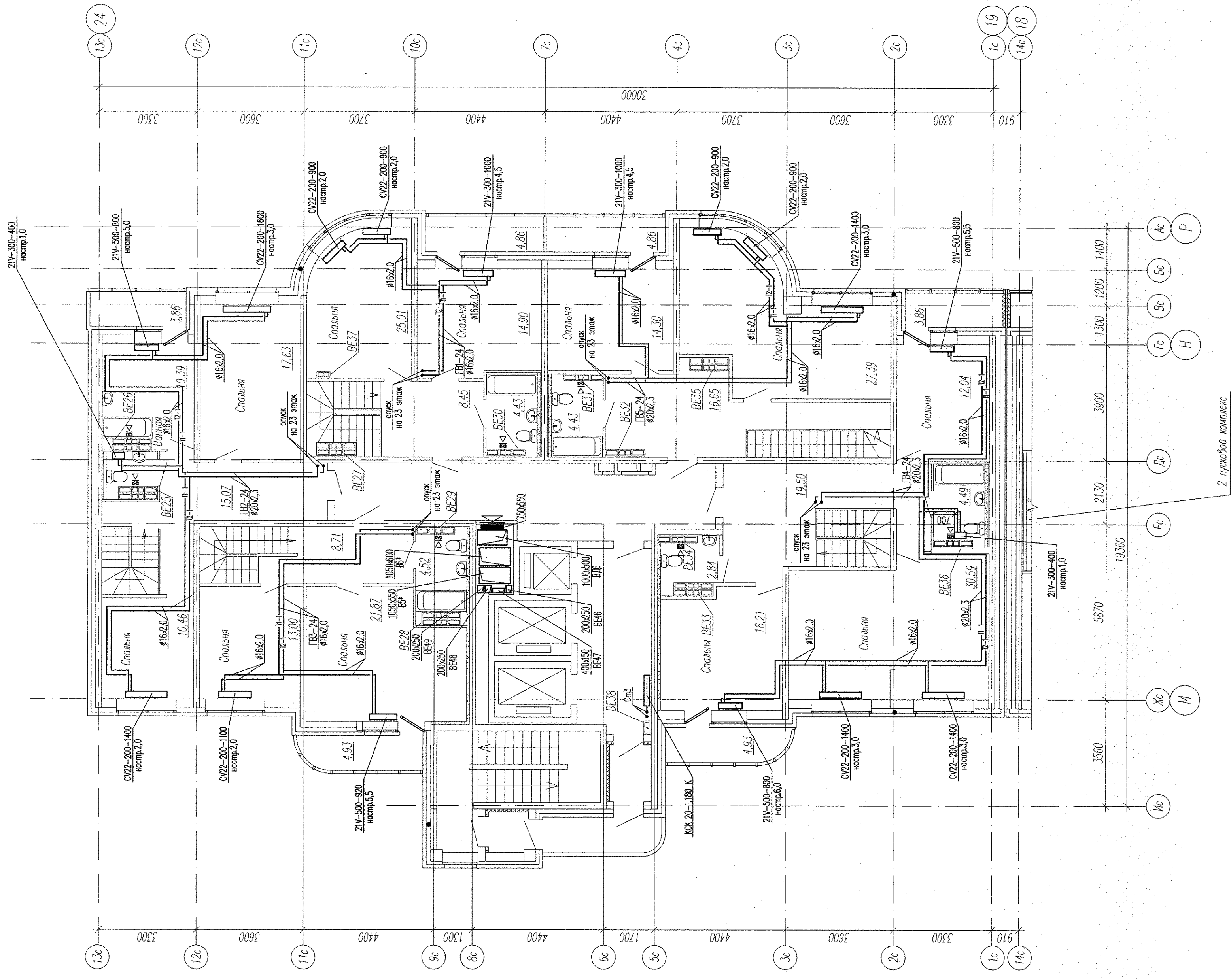
План 24 этажа
