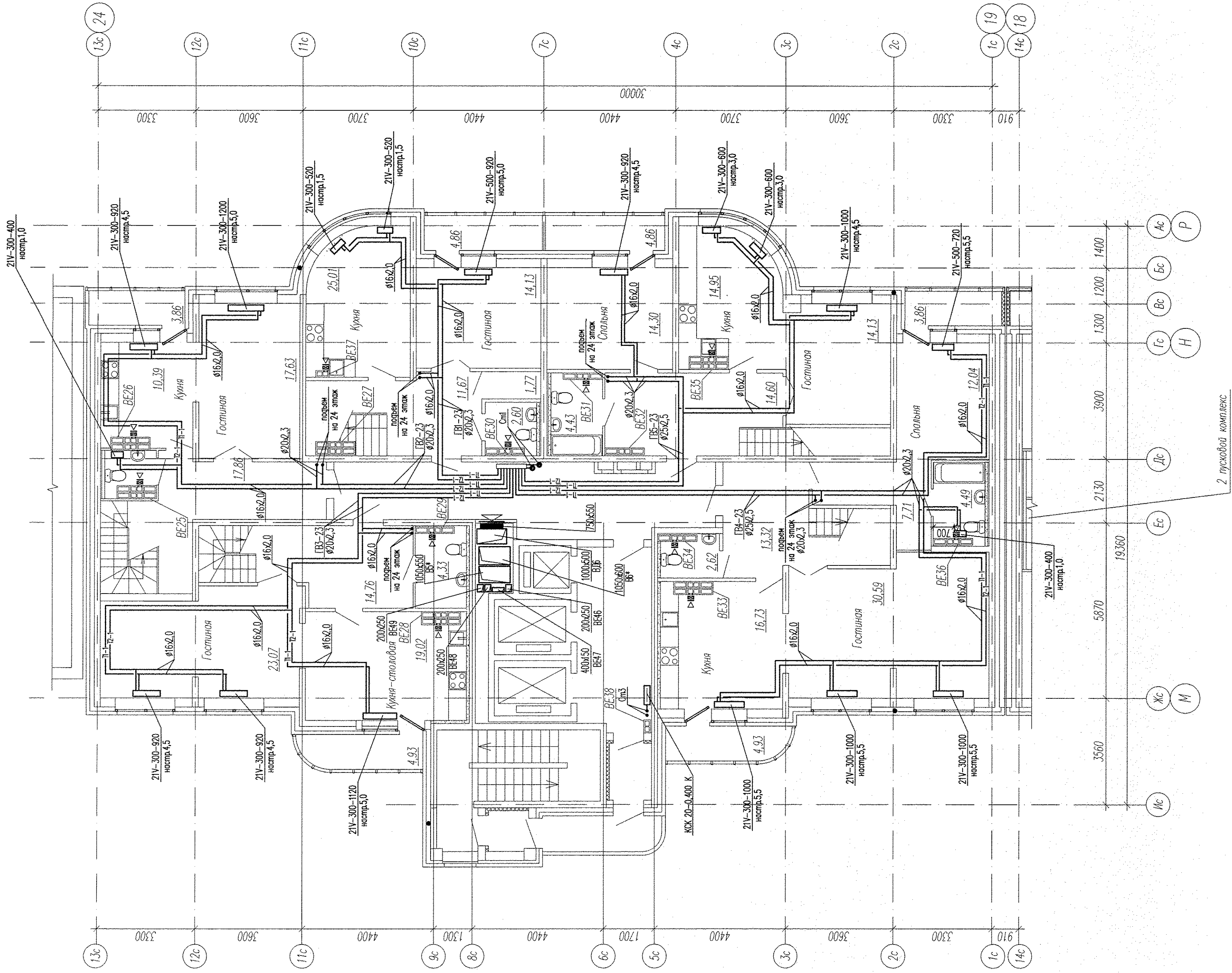
План 23 этажа
